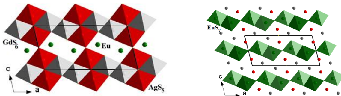
Рис. 2. Перспективные проекции [010] структуры соединения \text{EuGdAgS}_3
