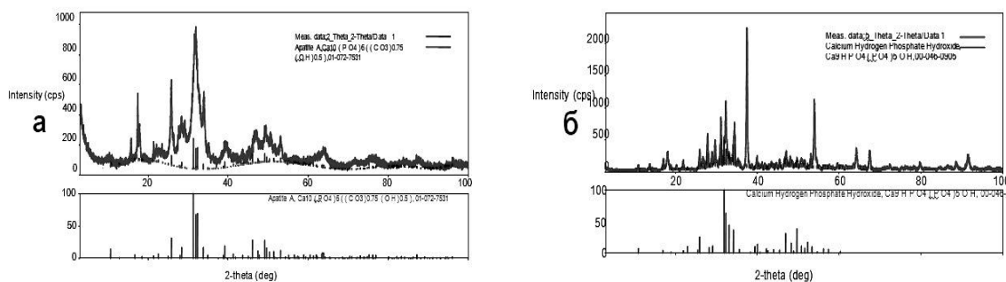
Рис. 1. Рентгенограммы порошков ГА, полученных в синтезах 1 (а) и 2 (б)
