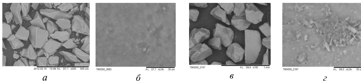
Рис. 1. Микрофотографии поверхности Силохрома С–120 до (а, б) и после (в, г) модифицирования ацетилацетонатом никеля
