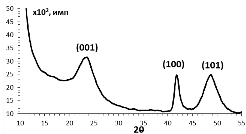
Рис. 1. Рентгенограмма \text{Ni}(\text{OH})_2/\text{Kemerit} композита, содержащего 40 масс.% \text{Ni}(\text{OH})_2
