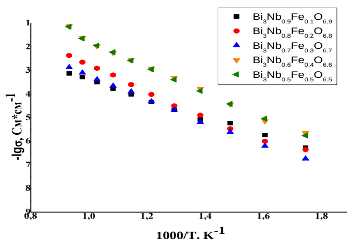
Рис. 2. Температурные зависимости электропроводности \text{Bi}_3\text{Nb}_{1-x}\text{Fe}_x\text{O}_{7\pm\delta}
