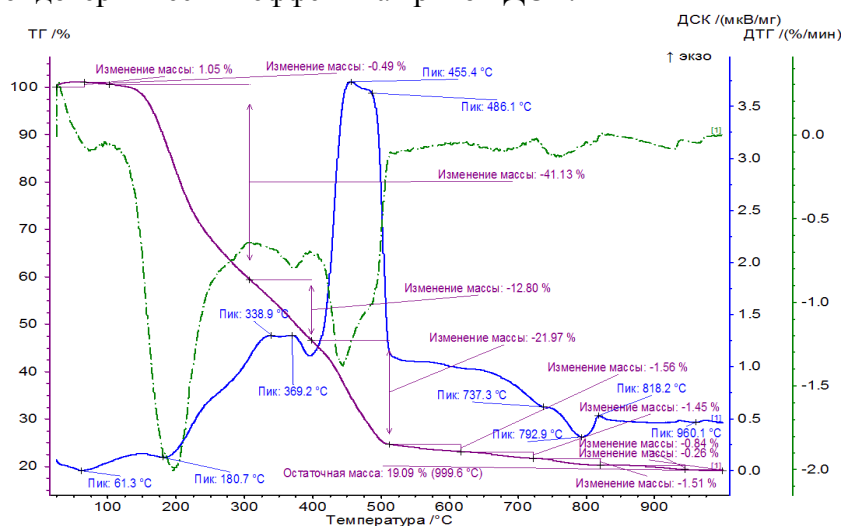
Рис.1. Термограмма прекурсора, полученного из гидроксида алюминия, карбоната бария и лимонной кислоты
