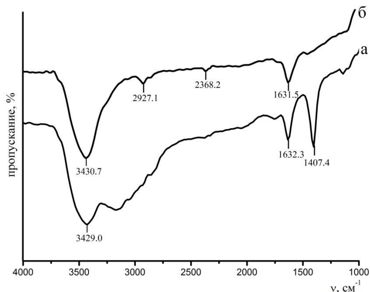
Рис. 2. ИК-спектры порошков SnO, полученных в микроволновых условиях с осадителями: а – \text{NH}_4\text{OH} ; б – \text{Na}_2\text{CO}_3
