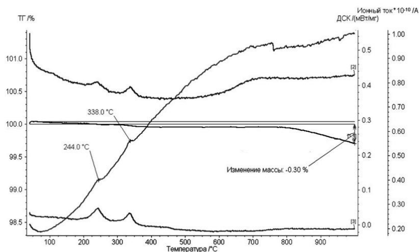
Рис. 1. Результаты ТГ/ДСК исследования для образца \text{La}_{0,9}\text{Bi}_{0,1}\text{Mn}_{0,9}\text{Ni}_{0,1}\text{O}_{3-\delta}
