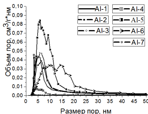
Рис. 3. Распределение пор по размерам
