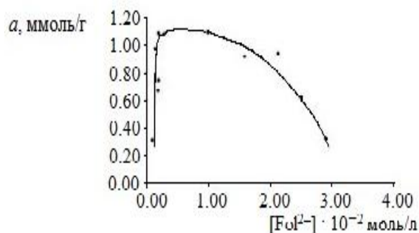
Рис. 1. Зависимость величины сорбции фолат-аниона от его равновесной концентрации в адсорбате
