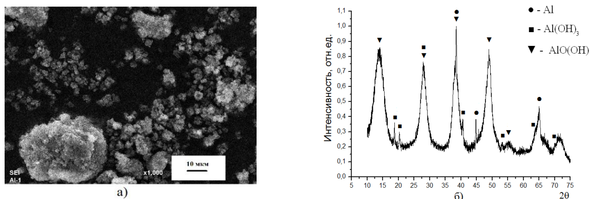
Рис. 1. Оксиды-гидроксиды алюминия: а – РЭМ-изображение; б – рентгенограмма
