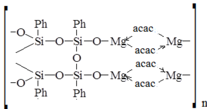
Рис. 1. Элементарное звено полимагнийфенилсилоксана
