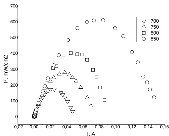
Рис. 1. Зависимости удельной мощности топливной ячейки от силы тока при различных температурах
