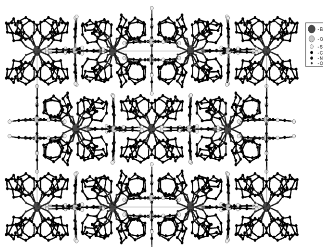
Рис.1. Общий вид структуры [\text{Er}(\epsilon\text{-C}_6\text{H}_{11}\text{NO})_8][\text{Cr}(\text{NCS})_6] . Атомы водорода не показаны
