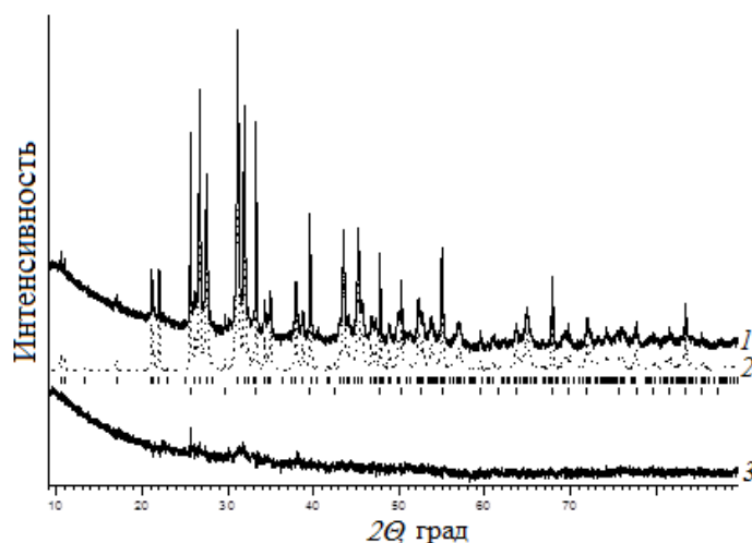
Рис. 1. Экспериментальная (1), расчетная (2) и разностная (3) дифрактограммы образца составов 2\text{EuS}:1\text{Gd}_2\text{S}_3:1\text{Ag}_{2-x}\text{S} после уточнения структуры методом МПР. Положения пиков основной фазы показаны штрихами
