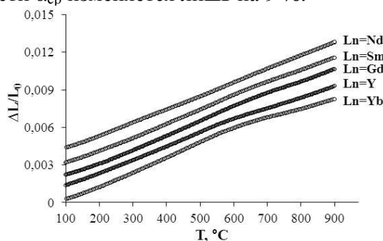
Рис. 1. Температурные зависимости линейного расширения на воздухе
