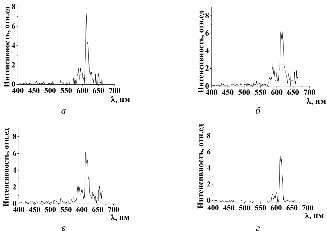
Рис. 1. Спектры люминесценции \text{Ca}_{0.99}\text{Eu}_{0.01}\text{Al}_2\text{O}_4 , полученного при мольном соотношении \text{Ca}^{2+}:\text{Al}^{3+}:\text{H}_4\text{Cit}:\text{Eg} равном: а) 1 : 2 : 3 : 0; б) 1 : 2 : 3 : 1,5; в) 1 : 2 : 6 : 0; г) 1 : 2 : 6 : 1,5
