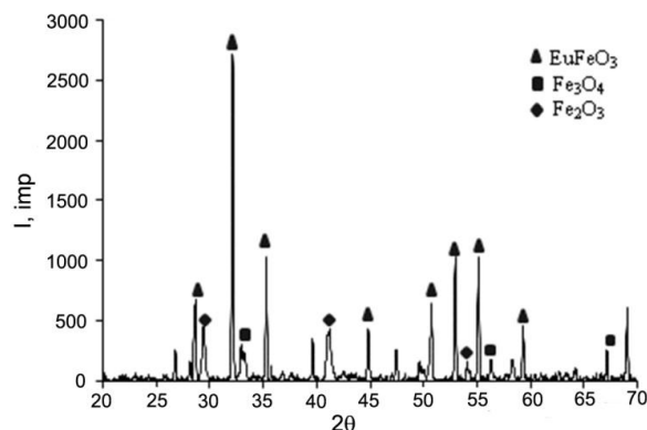
Рис. 2. Рентгеновская дифрактограмма образца \text{EuFeO}_3 после отжига в режиме 800 °С, 4 часа
