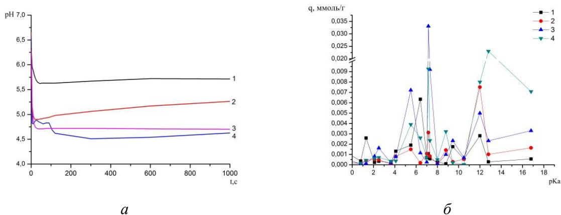
Рис.2. Кинетические кривые изменения pH (а) и распределение центров адсорбции индикаторов на поверхности сорбентов (б): 1 – SiO 2 , 2 – SiO 2 + Ni(AA), 3 – SiO 2 + Co(AA), 4 – SiO 2 + Cu(AA)
