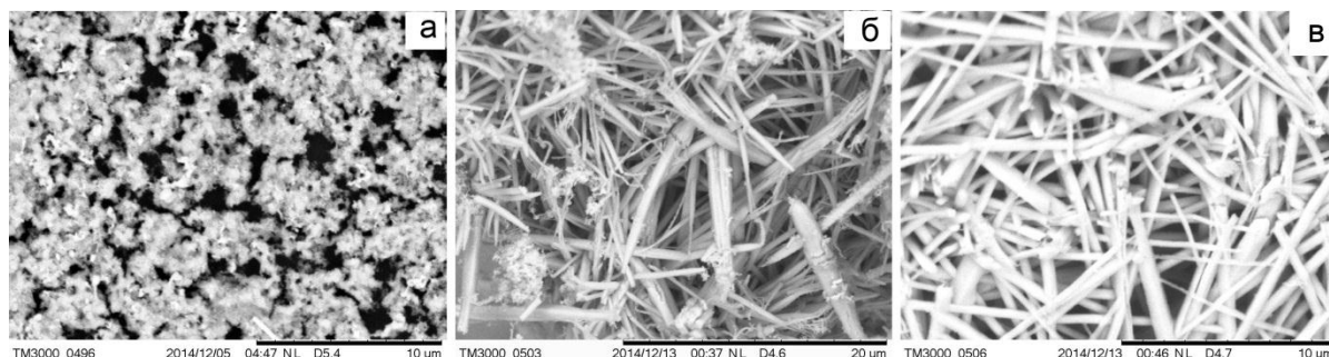
Рис. Микрофотография наночастиц соединения \text{Ag}_8\text{SnS}_6 при температурах а) 353 К; б) 403 К; в) 453 К
