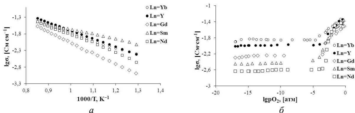
Рис. 2. Зависимости проводимости \text{BaCe}_{0.5}\text{Zr}_{0.3}\text{Ln}_{0.2}\text{O}_{3-\delta} материалов от температуры на воздухе (а) и парциального давления кислорода при 900 °С (б)
