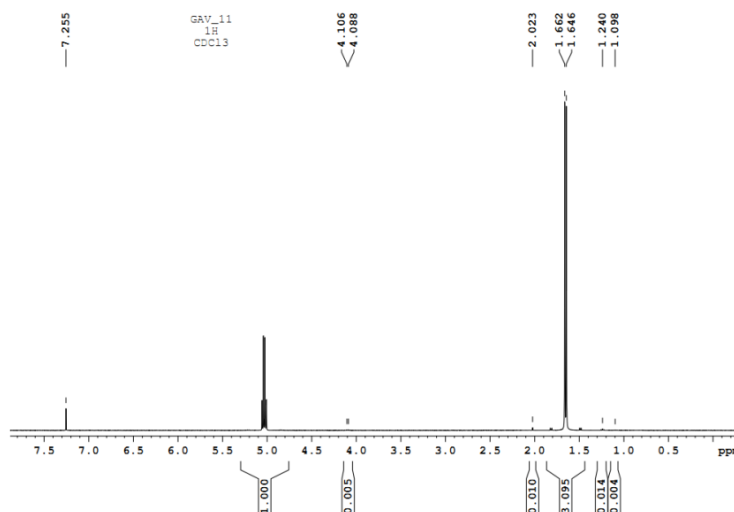
Рис. 1. Спектр ^1\text{H} ЯМР перекристаллизованного лактида, полученного из олигомера молочной кислоты с ММ ~600 г/моль (растворитель \text{CDCl}_3 )
