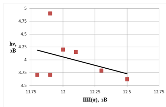
Рис. 2. Зависимость 1 для комплексов альдегидов и кетонов от потенциалов ионизации \pi системы
