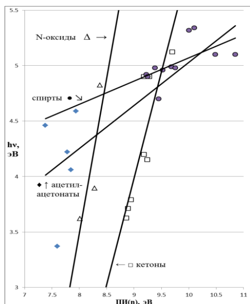
Рис. 1. Зависимость энергий полос переходов с переносом заряда от вертикальных потенциалов
