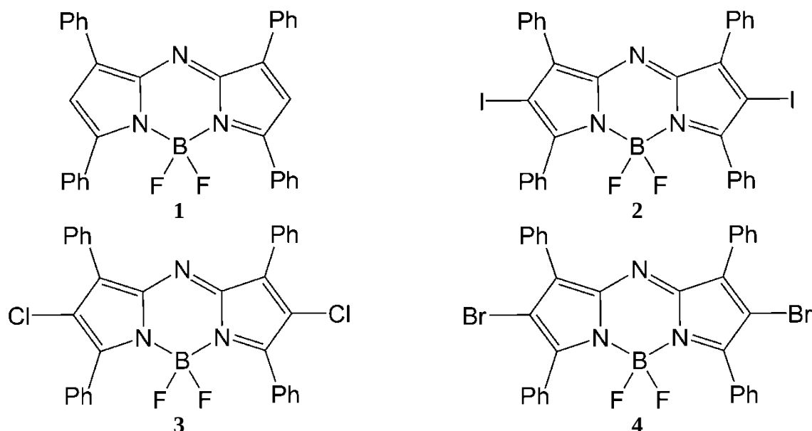
Рис. 1. Структурные формулы и обозначения: 1 – (Ph) 4 -N-BODIPY; 2 – I 2 (Ph) 4 -N-BODIPY; 3 – Cl 2 (Ph) 4 -N-BODIPY; 4 – Br 2 (Ph) 4 -N-BODIPY
