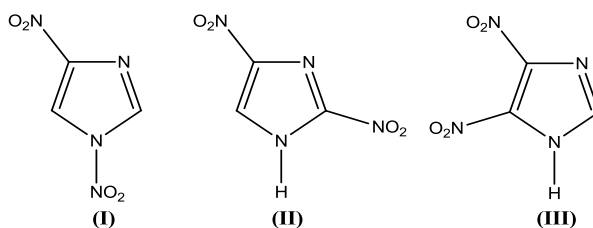
Рис. 1. Динитроимидазолы: 1,4-динитроимидазол (I), 2,4-динитроимидазол (II), 4,5-динитроимидазол (III)
