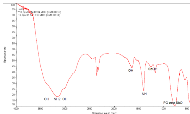
Рис.2. ИК-спектр ФСКК
