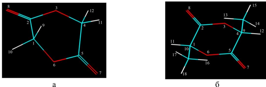
Рис.2. Модели молекул гликолида (а) и лактида (б)
