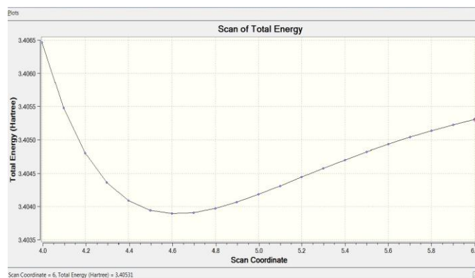
Рис. 1. Энергетическая зависимость адсорбционного взаимодействия 1,2-ди-(феноксифенил)-2 цианоэтилена с УНТ (6,6)
