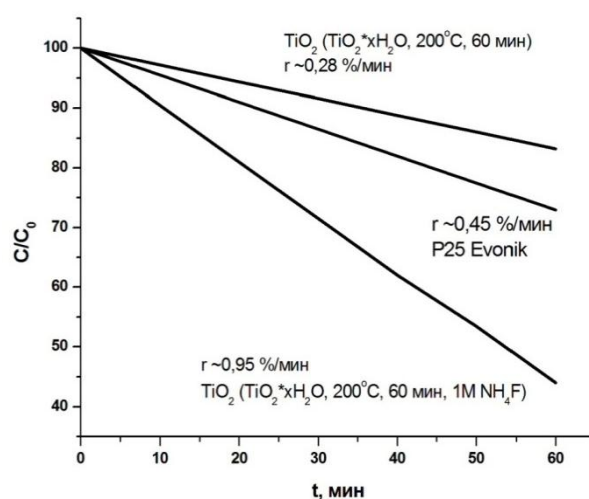
Рис. 1. Зависимость концентрации красителя фиолетового кристаллического от времени
