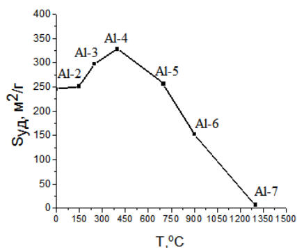
Рис. 2. Зависимость величины S_{уд} от T_{то} .
