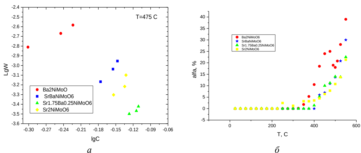
Рис.1. Зависимости скорости реакции окисления метана от его концентрации (а), температурные зависимости степени превращения метана (б)
