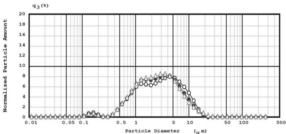
Рис. 1. График распределения частиц по размерам \text{LaNbO}_4
