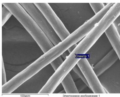
Рис. 1. СЭМ – изображение образца сорбента
