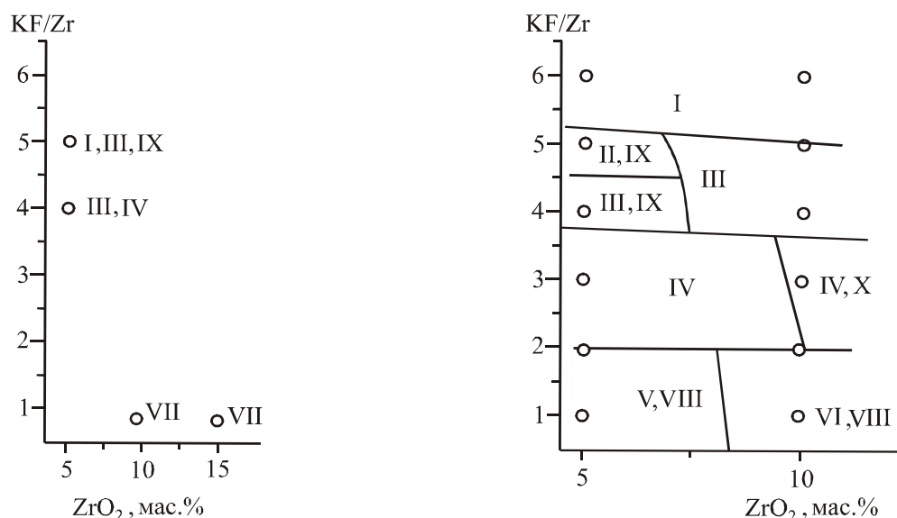
Рис. Поля образования фаз, м.о. C_2O_4/Zr а – 1, б – 2. Круги – экспериментальные точки. Обозначения полей: I – K_3ZrF_5C_2O_4 , II – фаза x, III – K_2ZrF_4C_2O_4 \cdot 2H_2O , IV – KZrF_3C_2O_4 \cdot 3H_2O , V – K_{0.5}ZrO_{0.25}F_2C_2O_4 \cdot 2H_2O , VI – K_2Zr_3O_{2.5}F_9 \cdot 7H_2O , VII – Zr_4O_3F_2(C_2O_4)_4 \cdot 2H_2O , VIII – рентгеноаморфные фазы, IX – KH_3(C_2O_4)_2 \cdot 2H_2O [5, карты 1-789, 14-845], X – KZrOF_3 \cdot 2H_2O
