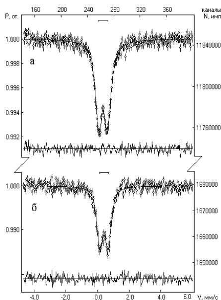
Рис. 2. Мёссбауэровские спектры образцов сорбентов: а – ионита Lewatit TP 260; б – новый сорбент (оба в Fe 3+ –форме)
