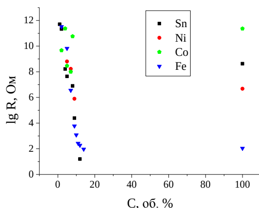
Рис. 1. Зависимость сопротивления пленок ППК с добавками наночастиц Fe, Co, Ni и Sn от концентрации наночастиц, T = 300 К
