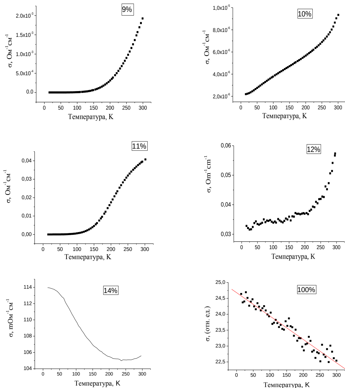
Рис.2. Зависимости проводимостей от температуры T пленок PPX + Fe с концентрацией наночастиц 9–100 об. %
