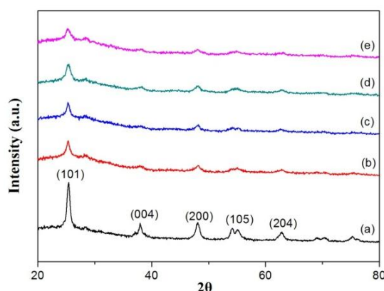
Fig. 2. XRD patterns of (a) \text{TiO}_2 , (b) VT1, (c) VT2, (d) VT3, and (e) VT4 samples after calcination
