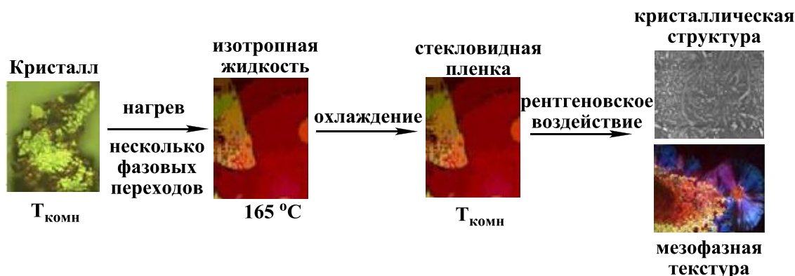
Рис. 4. Графическое представление последовательности превращения образца 4-((4-(N,N-дибутиламино)фенил)дiazенил)дифенил-2,3',4'-трикарбонитрила при комнатной температуре, нагреве, охлаждении и рентгеновском воздействии
