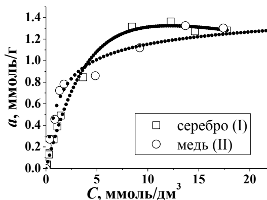
Рис. 1. Экспериментальные и теоретически рассчитанные по модели Редлиха-Петерсона изотермы сорбции серебра(I) и меди(II) СЭХ 1,0. Масса сорбента 0,0200 г. Аммиачно-ацетатный буферный раствор pH = 6,5; T = 298±2 К
