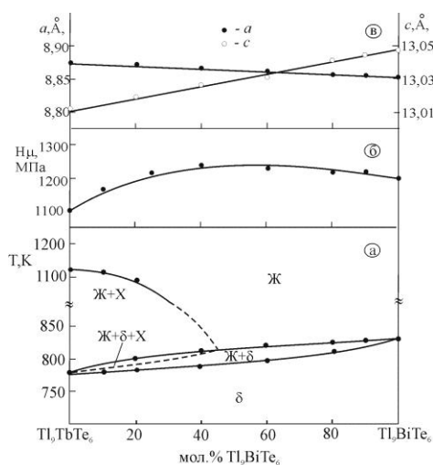
Рис. Фазовая диаграмма системы \text{Tl}_9\text{TbTe}_6 - \text{Tl}_9\text{BiTe}_6 (а), зависимости микротвердости (б) и параметров кристаллической решетки (в) от состава
