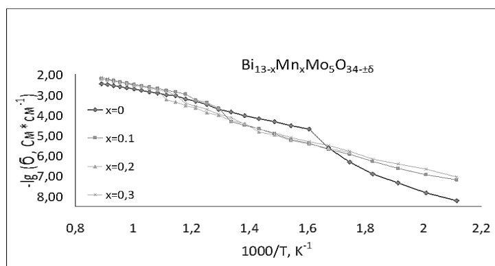
Рис. 2. Температурные зависимости электропроводности для чистого и допированного молибдата висмута
