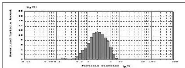
Рис. 1. График распределения частиц по размерам La_{1-x}Bi_xMn_{1-y}Cu_yO_{3\pm\delta}
