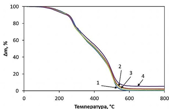
Рис. 1. Зависимость изменения массы образцов при нагревании для различных концентраций наполнителя, %: 1 – 0; 2 – 1; 3 – 5; 4 – 10
