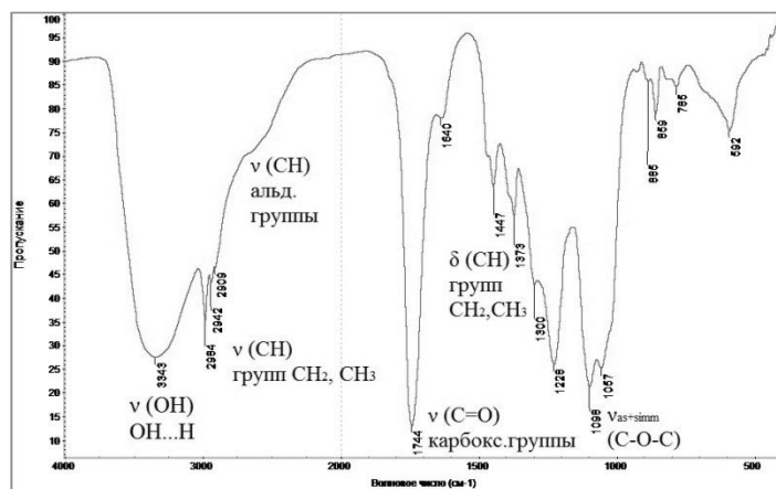
Рис. 3. ИК-спектр ЭГ, полученного из кальциевой соли ГК
