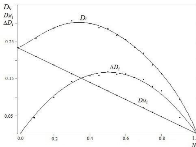
Рис. 1. Зависимость D_i , D_{M_i} и \Delta D_i от мольной доли лиганда в изомолярных растворах системы \text{Cr}(\text{NO}_3)_3 - \text{C}_6\text{H}_5\text{NO}_2 - \text{NaNO}_3 ( C_{\text{Cr}}^0 = C_{\text{Pic}}^0 = 0.05 моль/л, рН 2, V_{\text{общ}} = 10 мл, I = 0.3 , \lambda = 490 нм)
