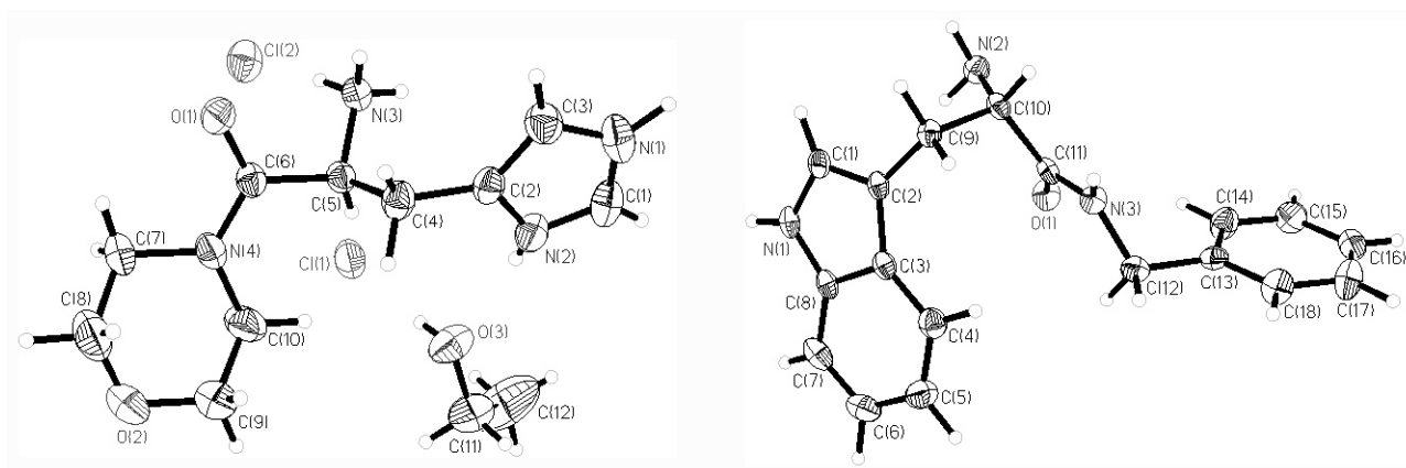
Рис. 1. Структура морфолида гистидина (слева) и бензиламида триптофана (справа)
