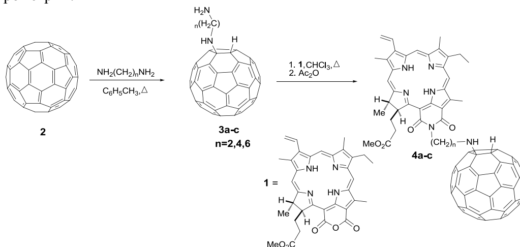
Рис. 1. Синтез конъюгатов циклических имидов хлорина p_6 и фуллерена C_{60} 4a-c
