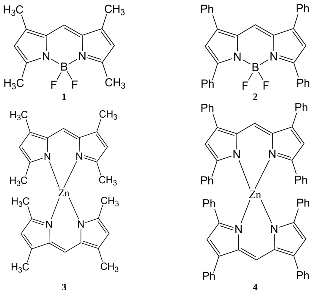
Рис.1. Структурные формулы соединений (1 – (CH 3 ) 4 -BODIPY, 2 – (Ph) 4 -BODIPY, 3 – Zn[(CH 3 ) 4 dpm] 2 , 4 – Zn[(Ph) 4 dpm] 2 )
