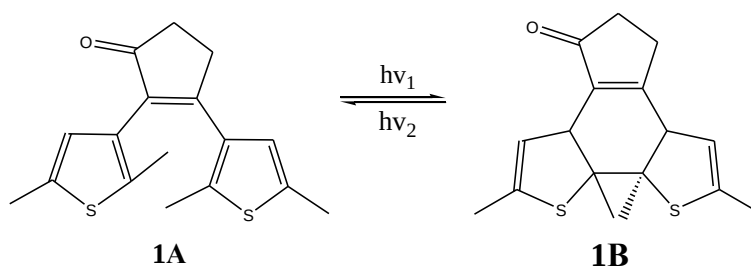
Рис. 2. Фотохромные реакции диарилциклопентенона ДМТЦ. Характерные длины волны фотоокрашивания и фотообесцвечивания 313 и 546 нм
