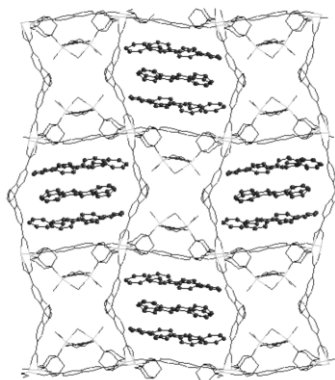
Рис. 1. Структура аддукта 1 (данные рентгеноструктурного анализа)
