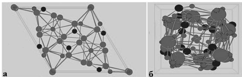
Рис. 2. Структуры гидроксиапатита (а) и пиррофосфата кальция (б) по результатам РФА образцов ГА
