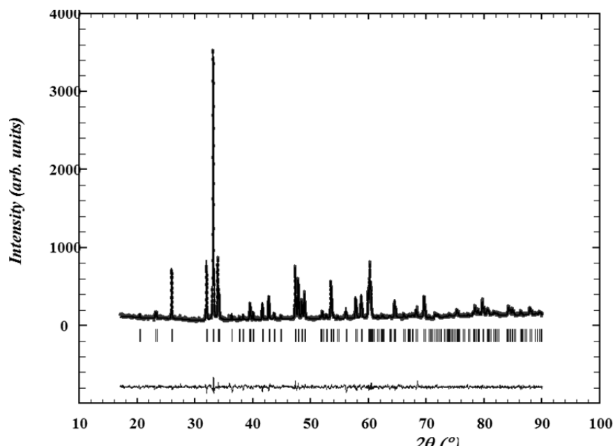
Рис. 1. Рентгенографические данные для YFeO_{3-\delta} , обработанные по методу Ритвелда: точки – экспериментальные данные; сплошная линия – теоретический спектр; сплошная нижняя линия – разница между экспериментальными данными и расчетным спектром
