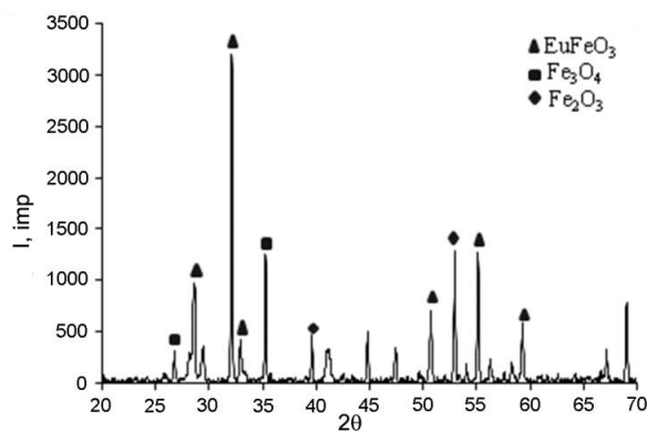
Рис. 1. Рентгеновская дифрактограмма образца \text{EuFeO}_3 после отжига в режиме 800 °С, 1 час
