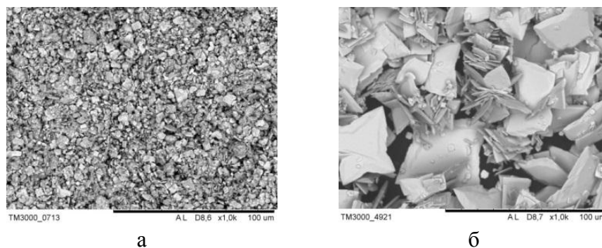
Рис. 1. Микрофотографии образцов, полученных с осадителями: а – \text{NH}_4\text{OH} ; б – \text{Na}_2\text{CO}_3
