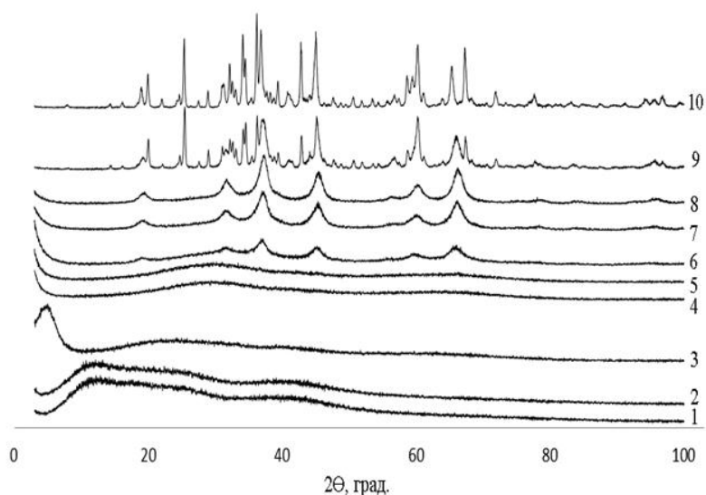
Рис.1. Дифрактограммы образцов, полученных при температурах °C: 1 – 100, 2 – 250, 3 – 350, 4 – 650, 5 – 700, 6 – 800, 7 – 900, 8 – 1000, 9 – 1100, 10 – 1200
