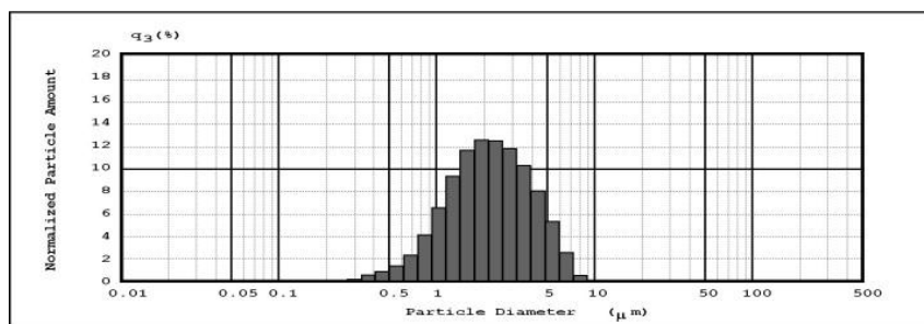
Рис. 2. График распределения частиц по размерам \text{La}_{0,9}\text{Bi}_{0,1}\text{Mn}_{0,5}\text{Ni}_{0,5}\text{O}_{3-\delta}
