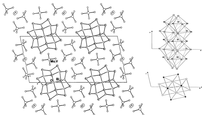
Рис. 1. Вид кристаллической структуры образцов керамики: \text{Bi}_{13-x}\text{Me}_x\text{Mo}_5\text{O}_{34\pm\delta}
