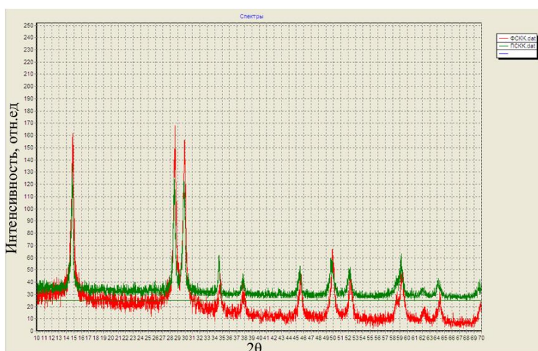
Рис.1. Сравнение спектров полисурьмяной кристаллической кислоты (ПСКК) [2] и фосфорносурьмяной кристаллической кислоты (ФСКК)
