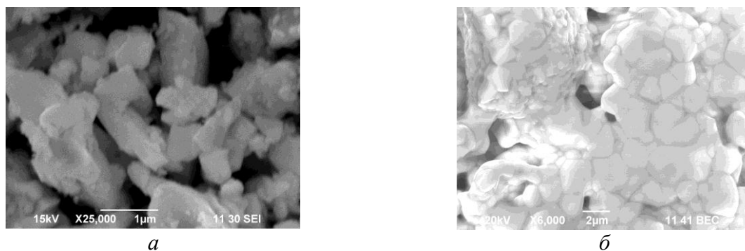
Рис. 1. Примеры СЭМ-изображений для ниобатов висмута: а) \text{Bi}_3\text{NbO}_7 ; б) скол керамического брикета \text{Bi}_3\text{Nb}_{0.85}\text{Zr}_{0.15}\text{O}_{7-\delta}
