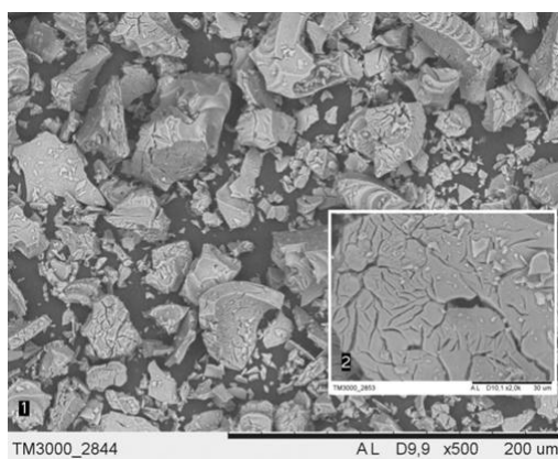
Рис. 2. Микрофотографии поверхности алюмината кальция-магния
