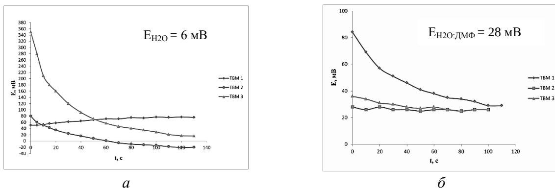
Рис. 1. Протолитические свойства тонковолокнистых материалов: а – в воде; б – в водно–ДМФА среде
