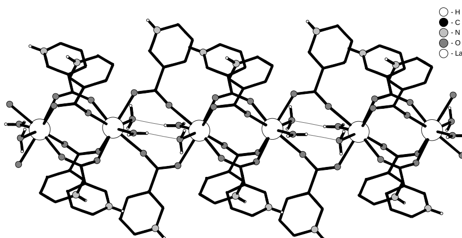
Рис. 2. Строение полимерной цепи в [\text{Nd}(\text{C}_5\text{H}_5\text{NCOO})_3(\text{H}_2\text{O})_2][\text{Cr}(\text{NCS})_6] \cdot \text{H}_2\text{O} . Внутримолекулярные водородные связи показаны пунктиром
