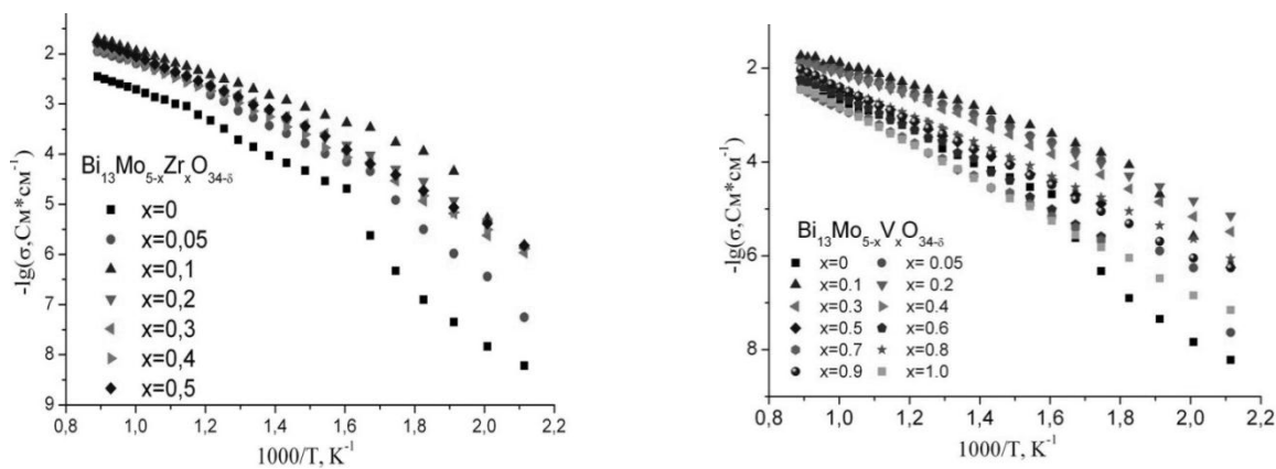
Рис. 2. Температурные зависимости электропроводности \text{Bi}_{13}\text{Mo}_{5-x}\text{Zr}_x\text{O}_{34\pm\delta} (а) и \text{Bi}_{13}\text{Mo}_{5-x}\text{V}_x\text{O}_{34\pm\delta} (б)
