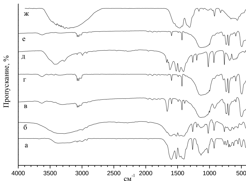
Рис. 2 ИК-спектры полученных фракций: а – фракция 1, б – фракция 2, в – фракция 3, г – фракция 4, д – \text{Mg}(\text{acac})_2 , е – ПФС, ж – \text{Mg}(\text{acac})_2 , прогретый при 250 °С
