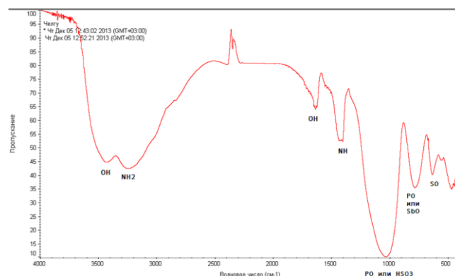
Рис.3. ИК-спектр серофосфорносурьмяной кислоты (СФСК)
