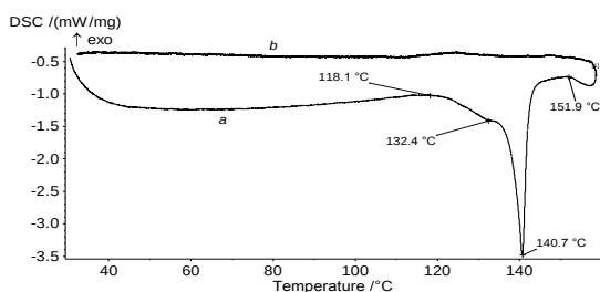
Рис. 1. ДСК первичного нагрева (а) и охлаждения (б) 4-((4-(N,N-дибутиламино)фенил)дiazенил)дифенил-2,3',4'-трикарбонитрила (10 °C мин -1 ).
