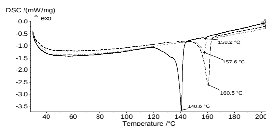
Рис. 2. ДСК трех последовательных нагревов азосоединения (первый – сплошная, второй – пунктирная, третий – точечная линия).
