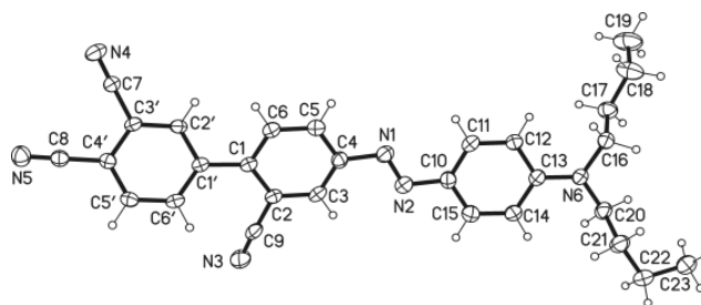
Рис. 3. Пространственная структура молекулы 4-((4-(N,N-дибутиламино)фенил)дiazенил)дифенил-2,3',4'-трикарбонитрила, определенная РСА
